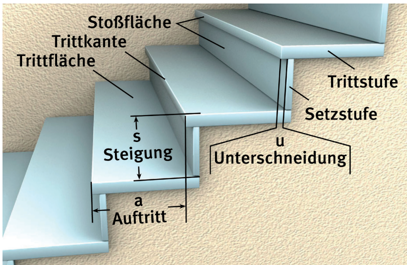
Abb. 1: Bezeichnung von Treppenteilen
