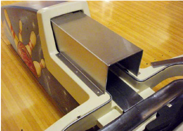
Abb. 39 Schutzmaßnahme: Schutztunnel
